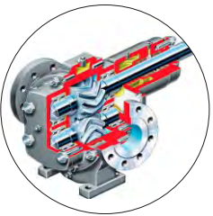
Bombas Engranajes Helicoidales Externos
