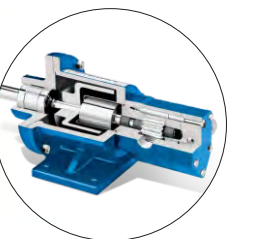
Bomba de Engranajes Externos
